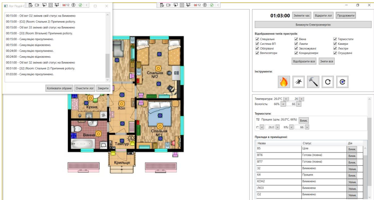
Рисунок 3.13. Відображення поточних станів температури, вологості та приладів в області приміщення «Спальня 2» з вікном «Лог Подій Системи»
